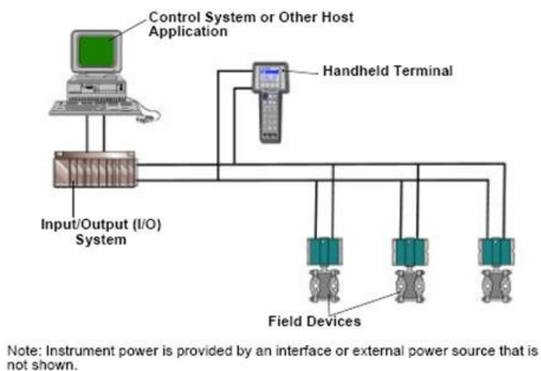
شکل ۸-۶ شبکه HART بصورت Multidrop
