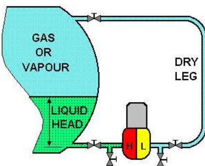
شکل ۴-۶ اتصال D.P.cell به مخزن سر بسته
