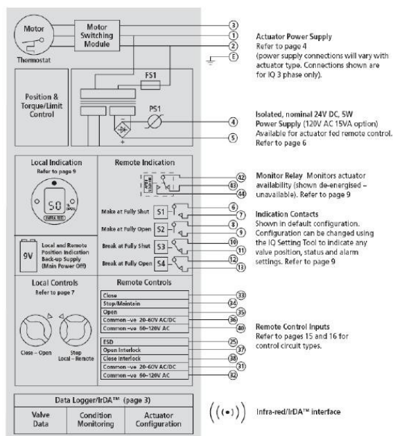
شکل ۳۰-۷ شماتیک مدار Rotork MOV
